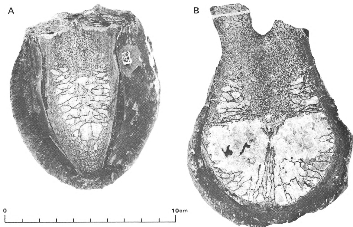
Figure 26. Internal structure of anterior caudal centra of Allosaurus fragilis (A, UUVP 4814) and Ceratosaurus sp. (B, UUVP 81).
